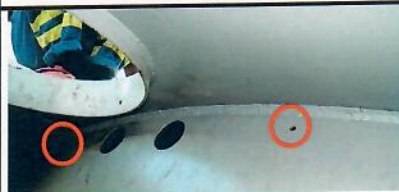
Détail intérieur n°5 Brise flot non étanche
