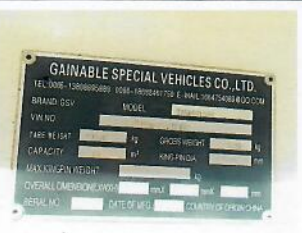
Plaque constructeur
